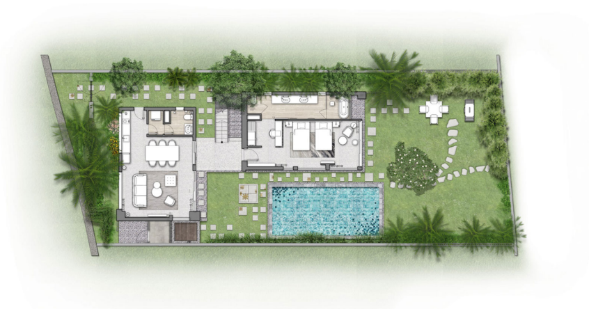
TẦNG TRỆT
